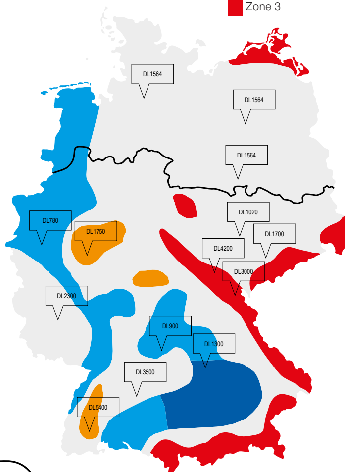
Beispiele örtlich erforderlicher DL-Klassen. Maßgebend sind Schneelastzone und Höhenlage. Auch die Dachform kann Einfluss haben. (hier Flachdach ohne Anhäufung)
