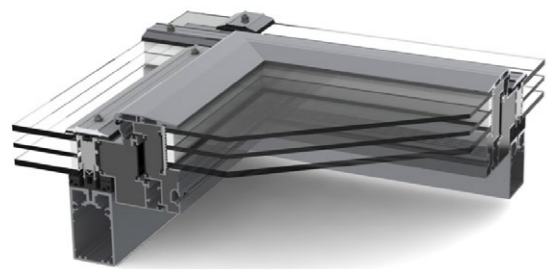
LAMILUX Lüftungsflügel PR60 Variante 1
